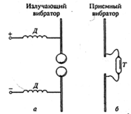
Рис. 178. Вибратор Герца
